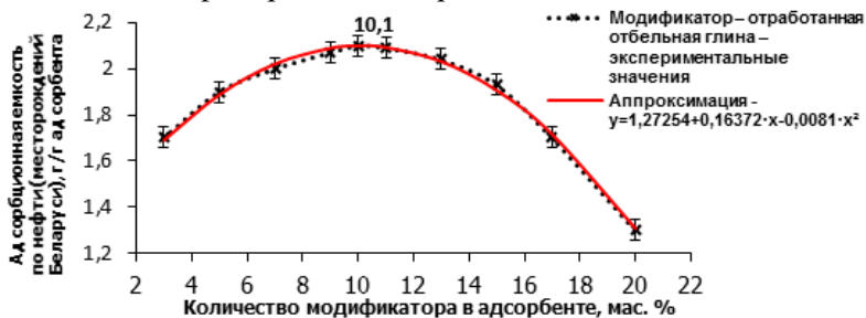
Рисунок –1. Нефтеемкость композиционного адсорбента на основе бentonитовой глины
