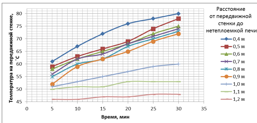
Рисунок – Динамика изменения температуры на передвижной стенке относительно расстояний от нетеплоемкой печи до передвижной стенке
