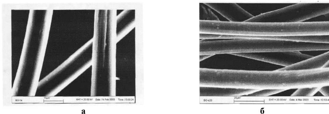
Рисунок – 1. Микроструктура поверхности: а – исходного, б - огнезащитного полиэфирного волокна
