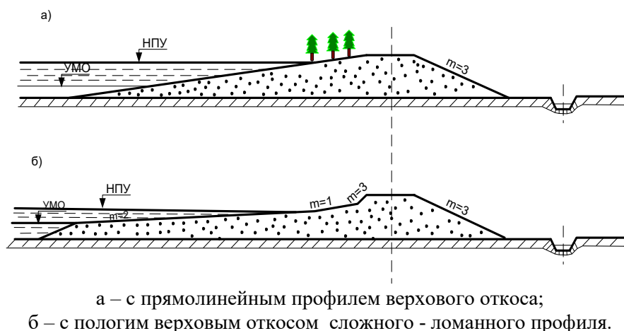
Рисунок – 1. Плотины распластанного профиля
