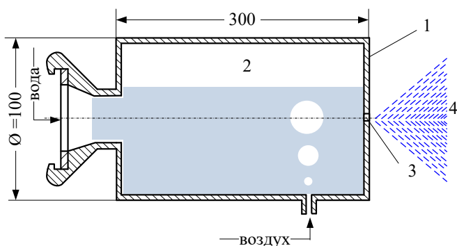
1 – корпус распылителя; 2 – свободный объем (ресивер); 3 – сопло; 4 – распыленная струя Рисунок – 1. Импульсная насадка на лафетный ствол
