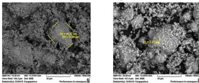
Рисунок – 2. Микрофотографии исходной и модифицированной бentonитовой глины
