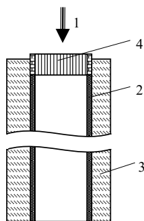
Рисунок – 2. Узел пиролиза: 1 – газовый поток, 2 – теплоизолированный канал, 3 – тепловая изоляция, 4 – устройство,
