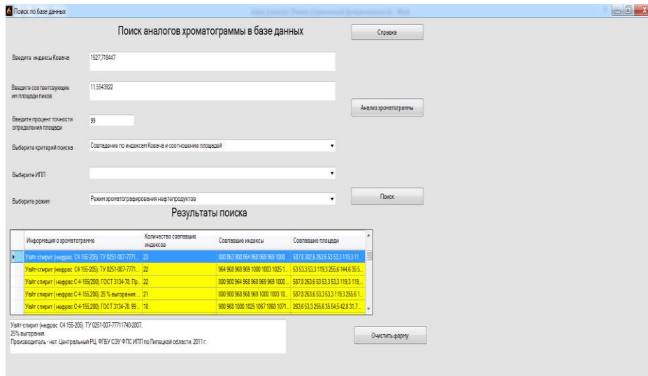
Рисунок – 2. Интерфейс программы поиска по базе данных хроматограмм
