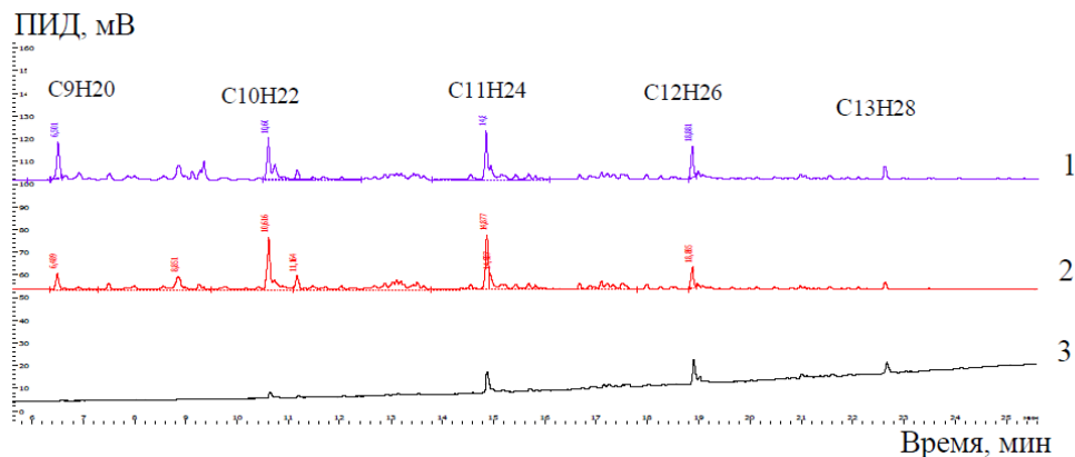
Рисунок – 1. Хроматограммы керосина осветительного ТУ 0251-015-57859009-2015: 1 – не подвергшегося термическому воздействию; 2 – со степенью выгорания 50 % (по масс.); 3 – со степенью выгорания 99 % (по масс.)
