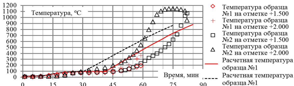
Рисунок –1. Экспериментальные и расчетные значения температуры образцов №1 и №2
