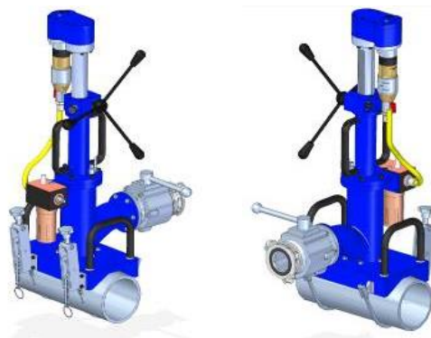
Рисунок –1. Устройство оперативной врезки интегрированное
