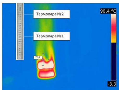
Рисунок – 2. Температурное поле потока пожаротушающей смеси на 5 секунде после сработки ГОА
