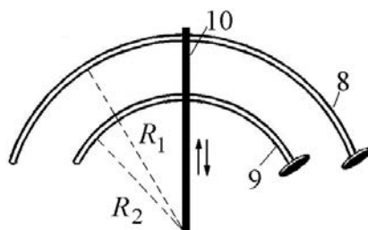
Рисунок – 2. Передача деформации измеряемого объекта на измерительные волокна
