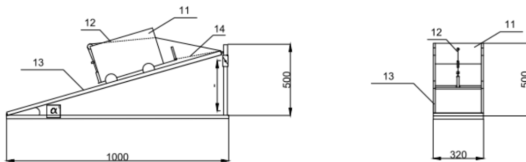
Рисунок – 3. Устройство для погружения каменной смеси
