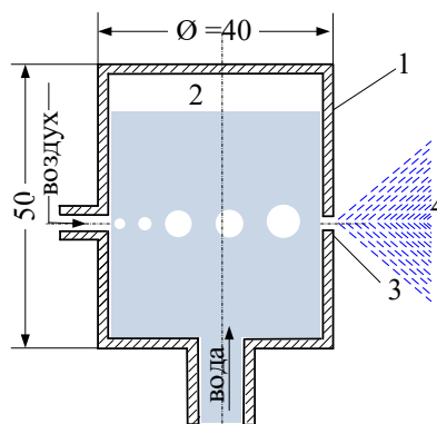
1 – корпус распылителя; 2 – свободный объем (ресивер); 3 – сопло; 4 – распыленная струя Рисунок – 1. Импульсная насадка на лафетный ствол
