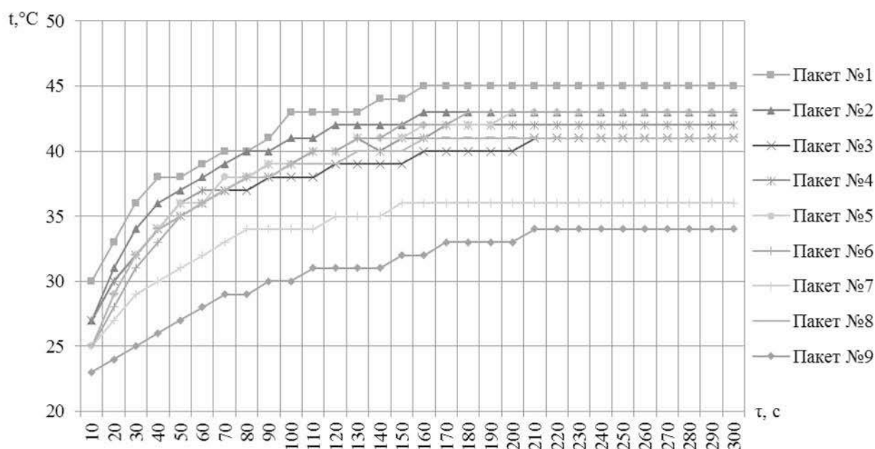
Рисунок 2. – Графики изменения температуры на внутренней поверхности материала, температура воды 70 \pm 5 °С
