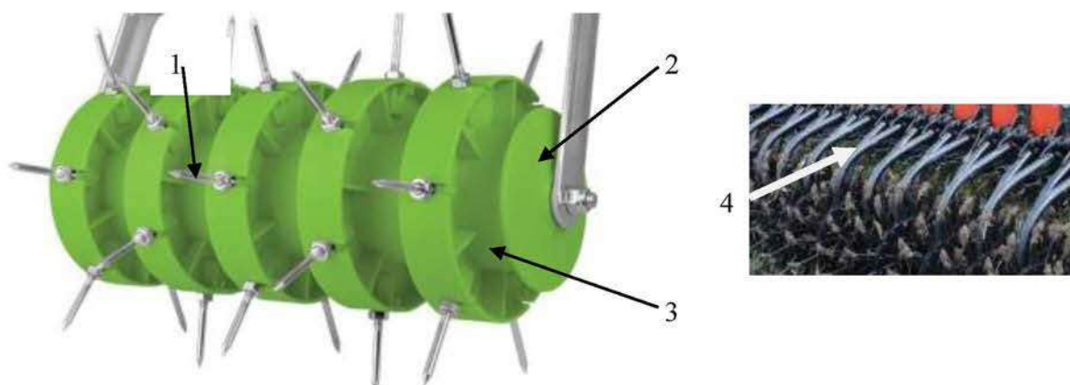
1 – выдвижные шипы, 2 – вал, 3 – пазы для снимающих слой ППР ножей, 4 – ножи
