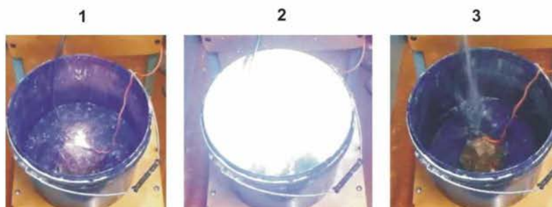
Рисунок 1. – Последовательные фазы частотного электрогидравлического воздействия на фрагмент железобетонной плиты находящейся в емкости с водой: 1 – начало процесса, 2 – максимальная фаза, 3 – финальная фаза
