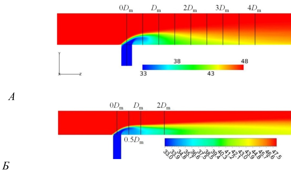
Рисунок 1 – Распределение осредненной температуры в срединном сечении тройникового соединения при отношении входных чисел Рейнольдса 5,76, полученное методом: а – LES [5]; б – RANS
