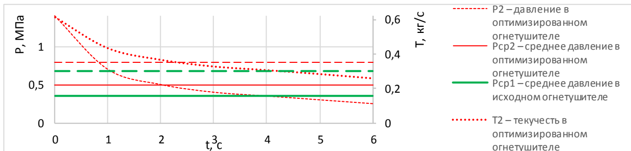
Рисунок 5 – Значение параметра давления перед насадком-распылителем
