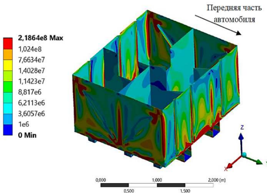
Рисунок 1. – Модель распределения полей эквивалентных напряжений по Мизесу в конструкции серийной цистерны пожарного автомобиля при движении по проселочной дороге с чередующимися неровностями и перепадами высот со скоростью 20–30 км/ч, Па
