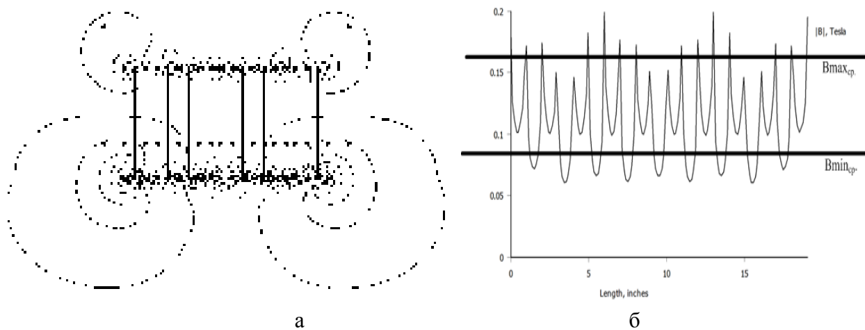
Рисунок – 4 Магнитный расчет уплотнения с немагнитными шайбами: а - картина магнитного поля; б - кривая распределения магнитной индукции в рабочей области
