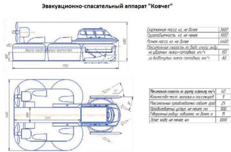
Рис. 2. Эвакуационно-спасательный аппарат «Ковчег» (КВЛ — конструктивная ватерлиния)
