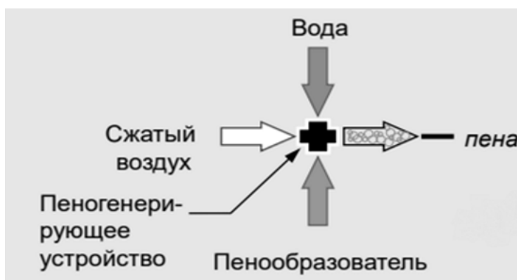
Рисунок 1 Схема установки генерирования пены компрессионным способом
