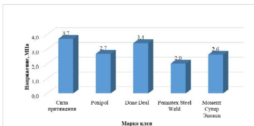
Рисунок 2 – Результаты эксперимента с алюминиевыми и стальными образцами
