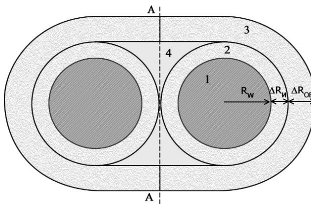
1 – медная жила, 2 – изоляция, 3 – оболочка кабеля, 4 – воздушный промежуток, AA – линия симметрии
